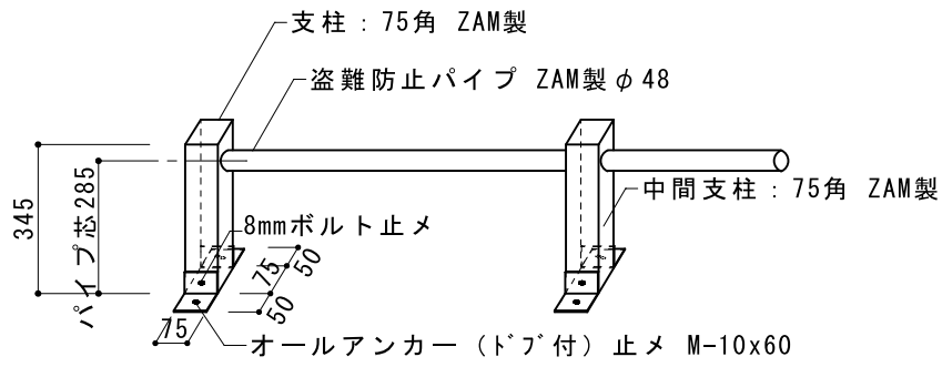
■ 姿図 S=1/20
