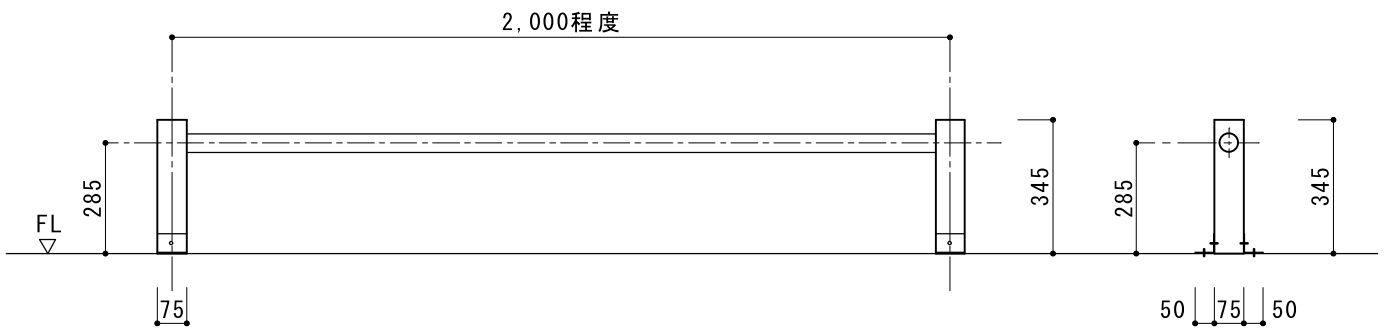
■ 正面図 S=1/20
