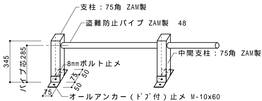
姿図 S=1/20
