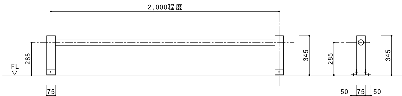
正面図 S=1/20
